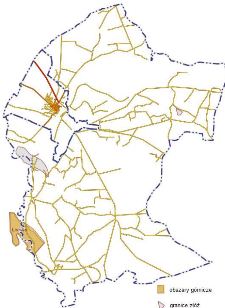
Ryc. 18. Obszary górnicze i granice złóż na terenie gminy Pyzdry
