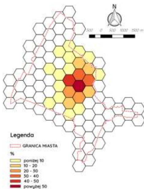
Ryc. 4. Koncentracja (% udział) występowania terenów zabudowy na obszarze miasta Pyzdry
