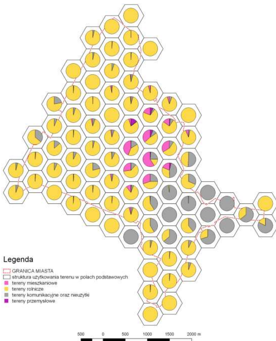
Ryc. 7. Zestawienie poszczególnych form użytkowania terenu w mieście dla każdego pola podstawowego w postaci wykresu kołowego
