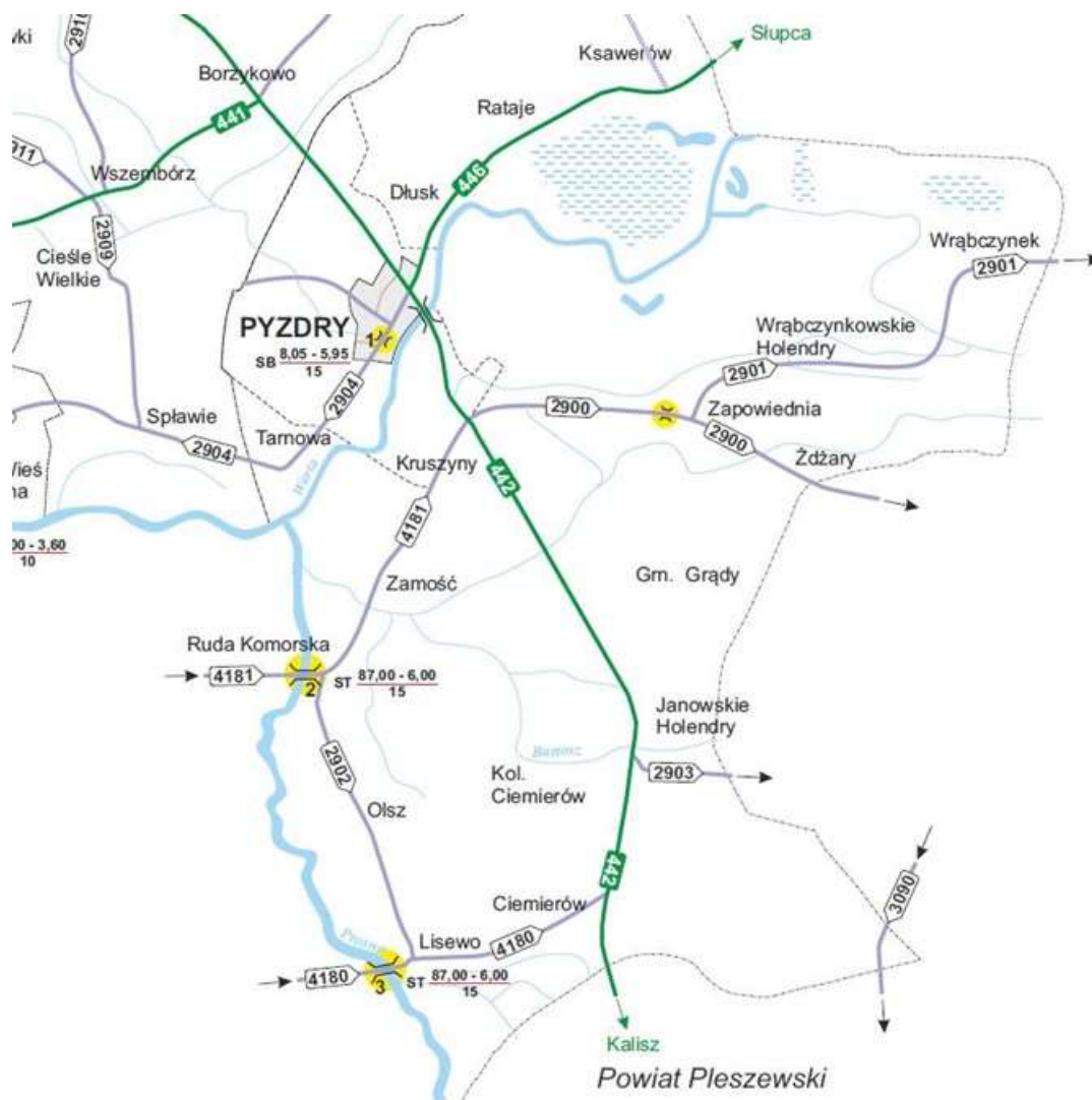
Ryc. 17. Gmina Pyzdry na tle sieci komunikacyjnej
